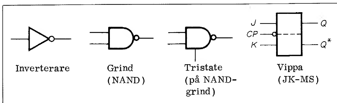
Fig 2.11 De fyra digitala "byggstenarna"
