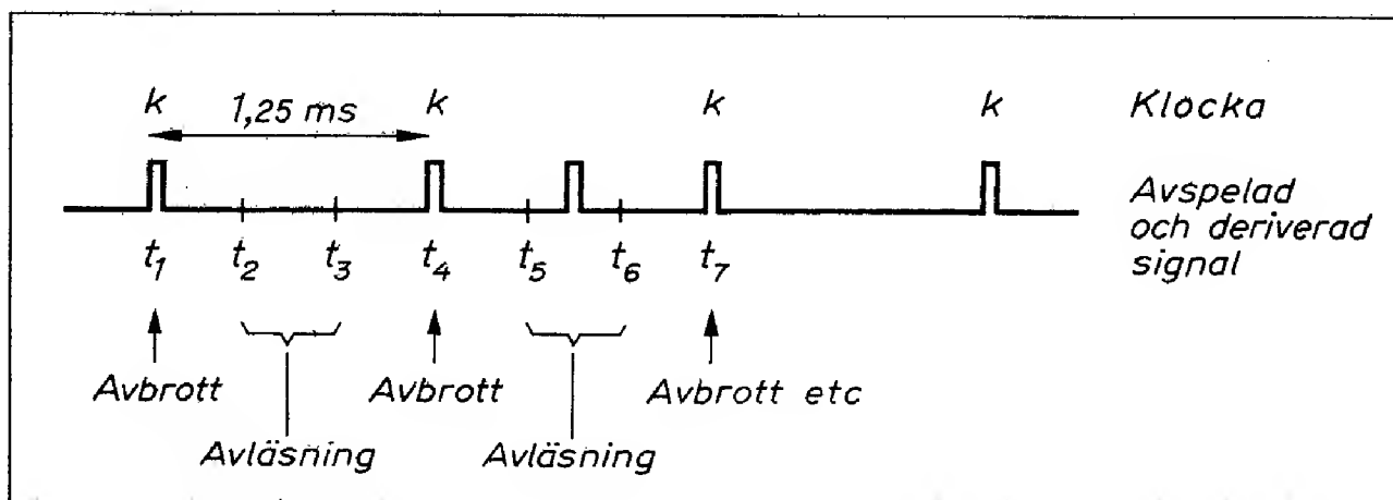
Fig 6.31 Hur ABC80 avkänner signalen från kassetbandspelaren
