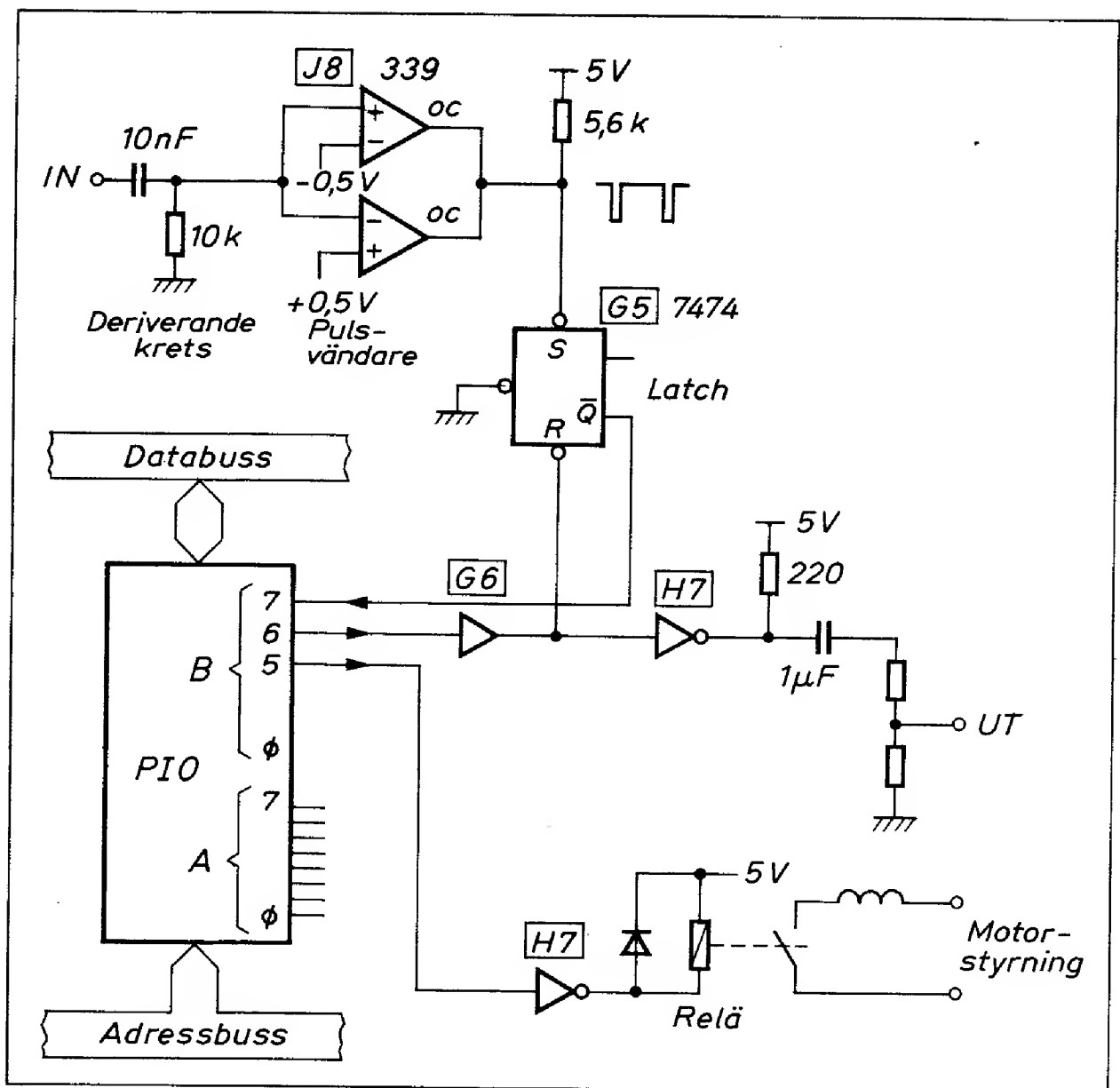
Fig 6.29 ABC80:s kassettinterface
