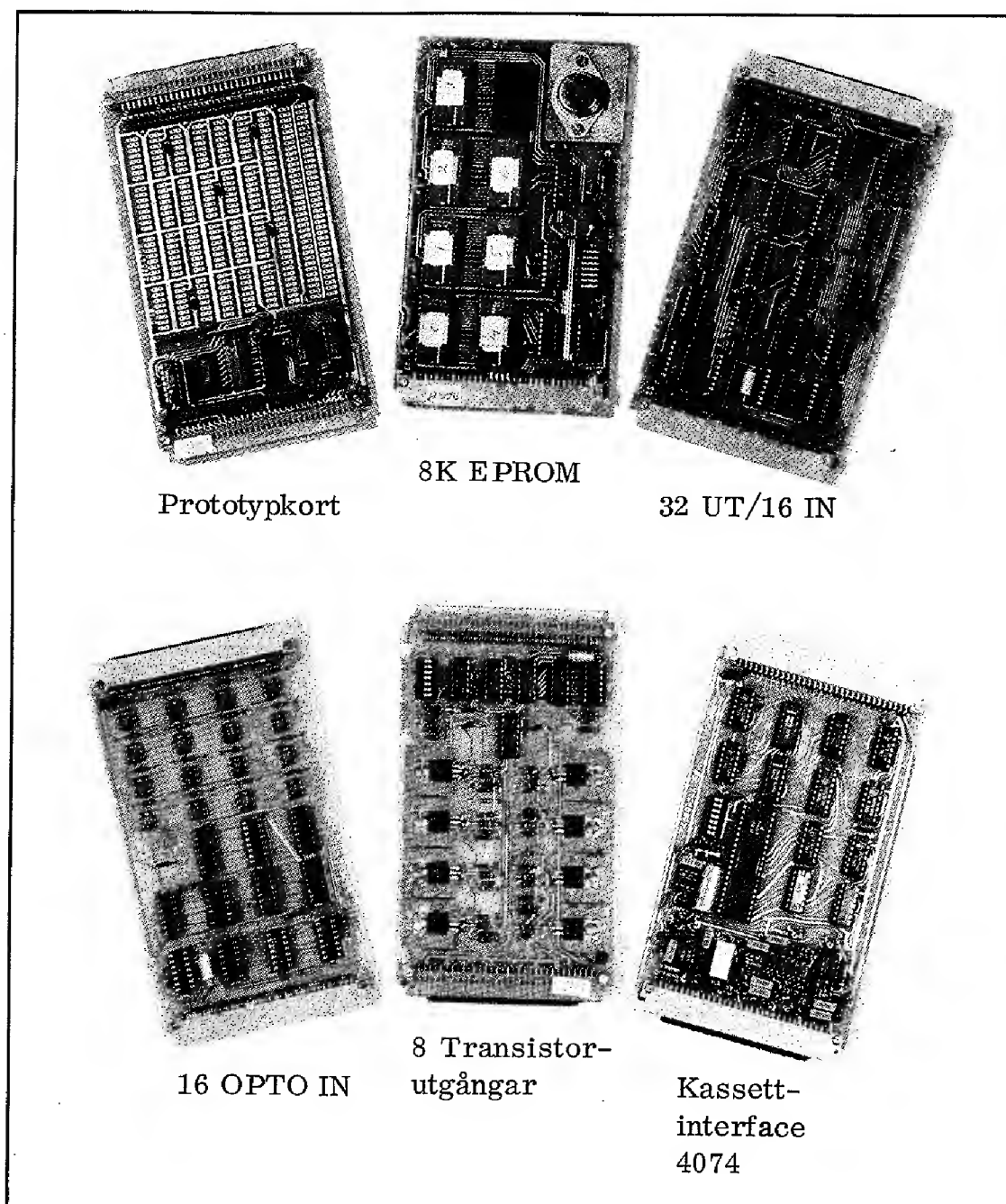
Fig 6.38 Exempel på Databoard-kort för ABC-bussen
