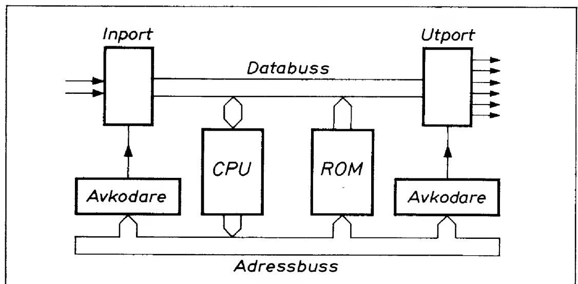
Fig 4.1 Enkel datorstruktur
