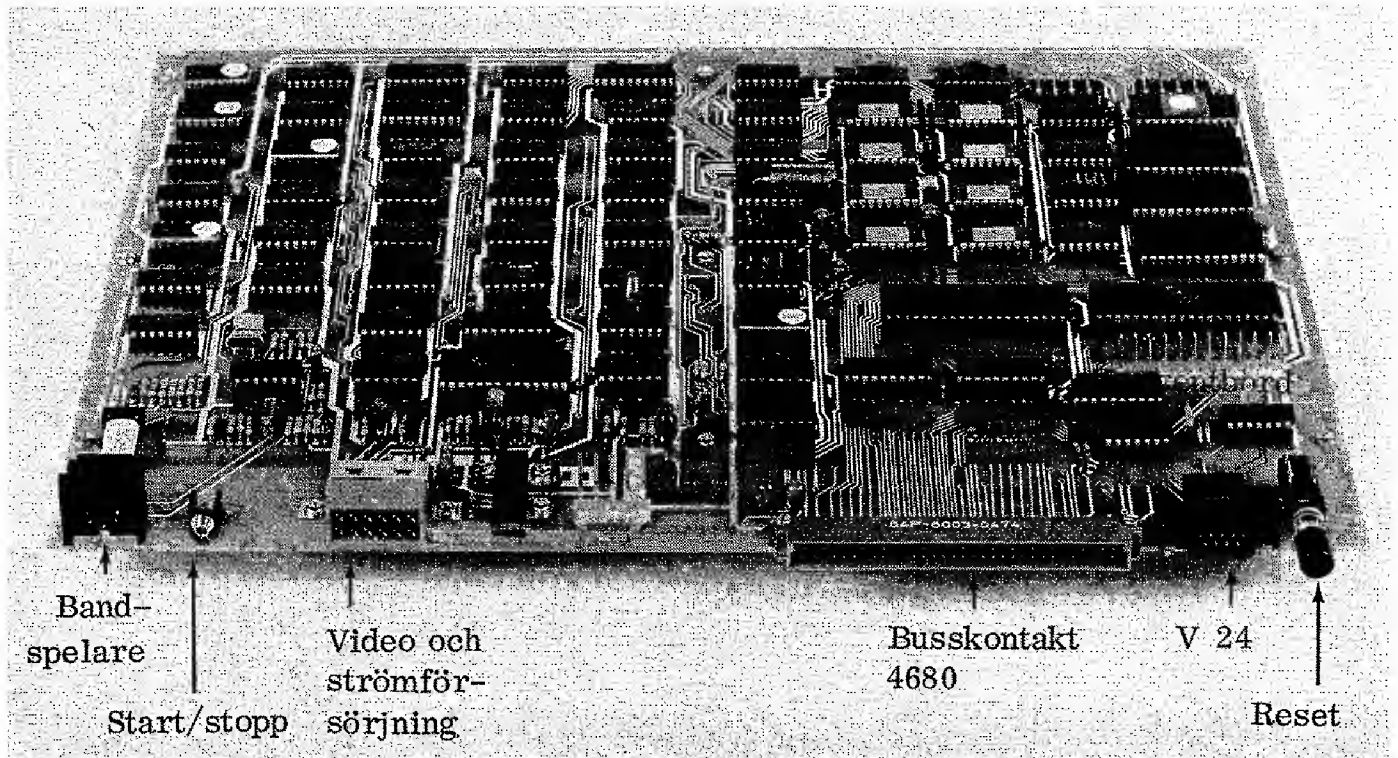
Fig 5.25 Uttagen på ABC80:s kretskort
