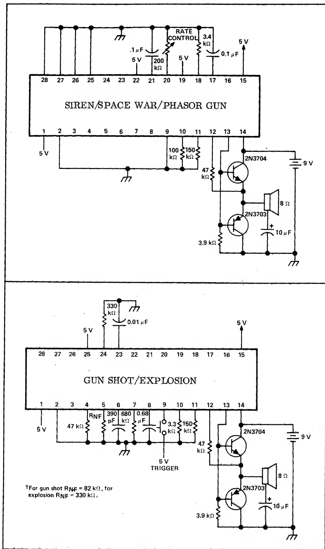
Fig 5.17 Exempel på ljudgenerering med krøtsen 76477
