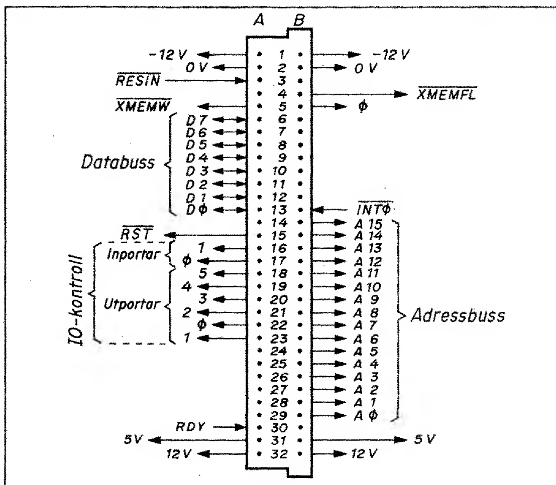
Fig 5.26 4680-kontakten i ABC80 och dess pinfunktioner
